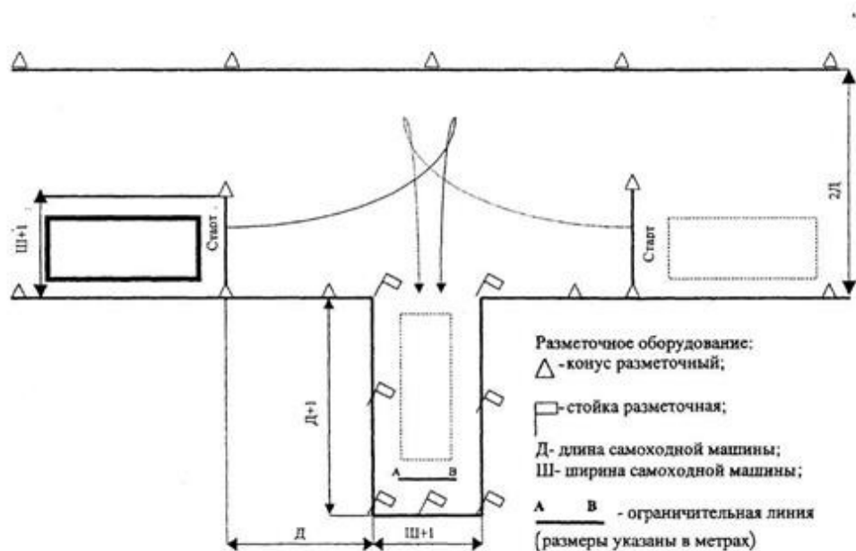
Рис. 6. Постановка самоходной машины в бокс задним ходом
