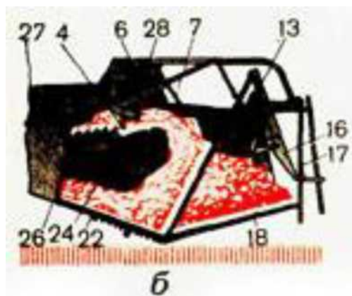
б, в- схема рабочего процесса заполнения копнителя и выгрузки
