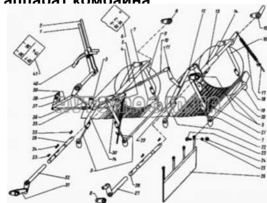
Рис. 10. Механизм регулировки подбарабья.
