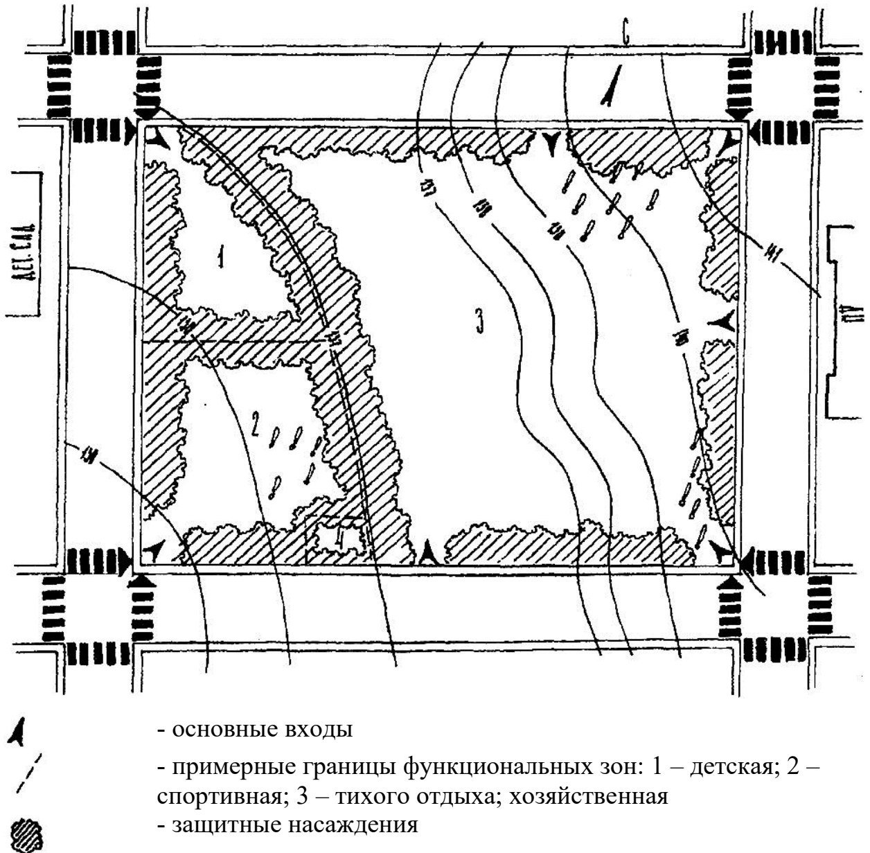
Рис. 2. 1-й этап эскиза
