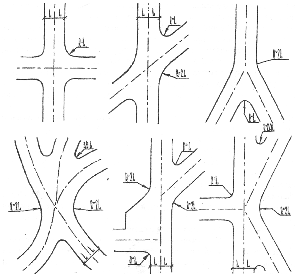
Рис. 5. Примеры пересечения парковых дорожек
