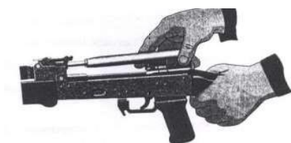
Рис. П.2.22. Отделение затворной рамы с затвором
