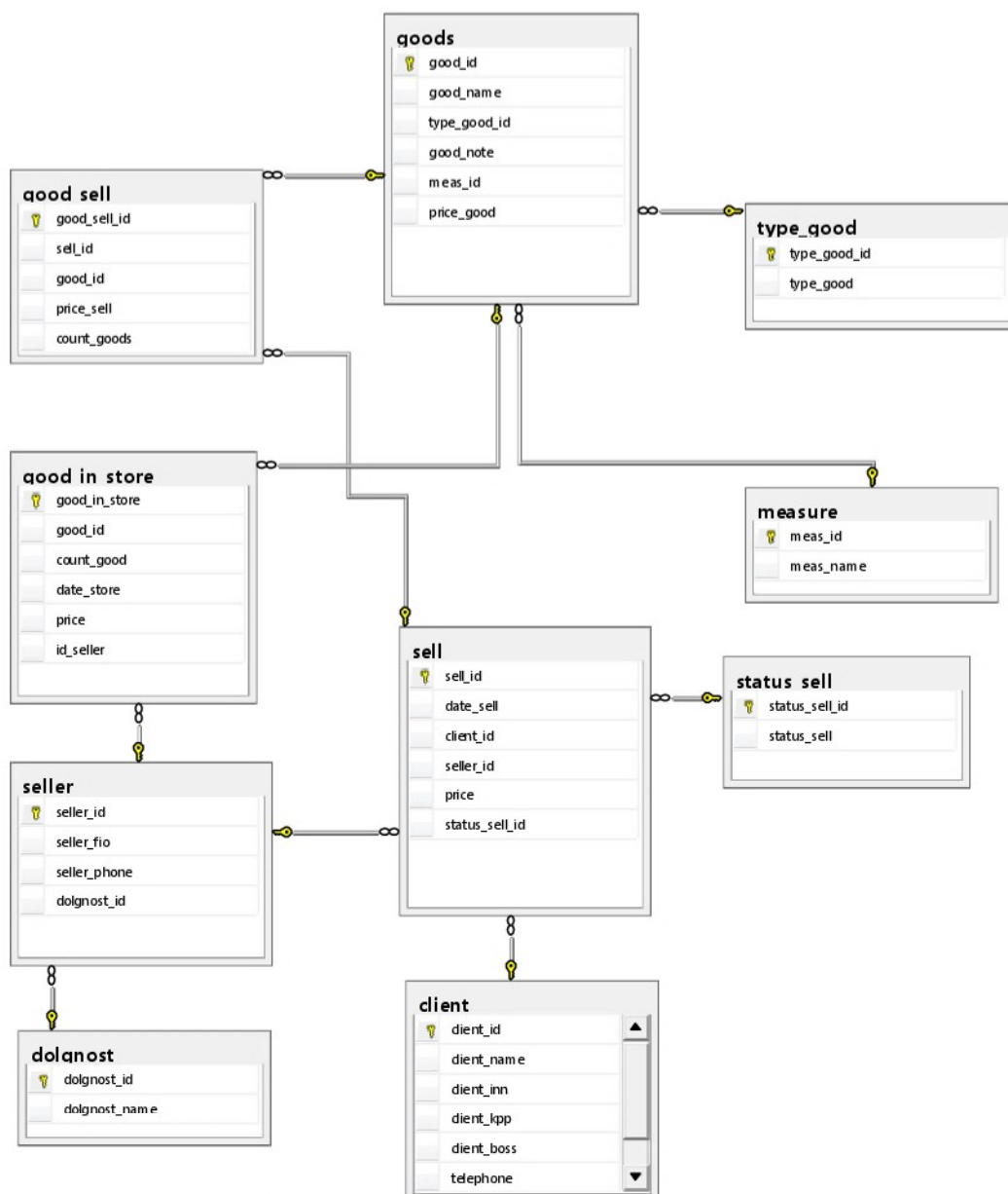
Рисунок 2.2 – Диаграмма базы данных
