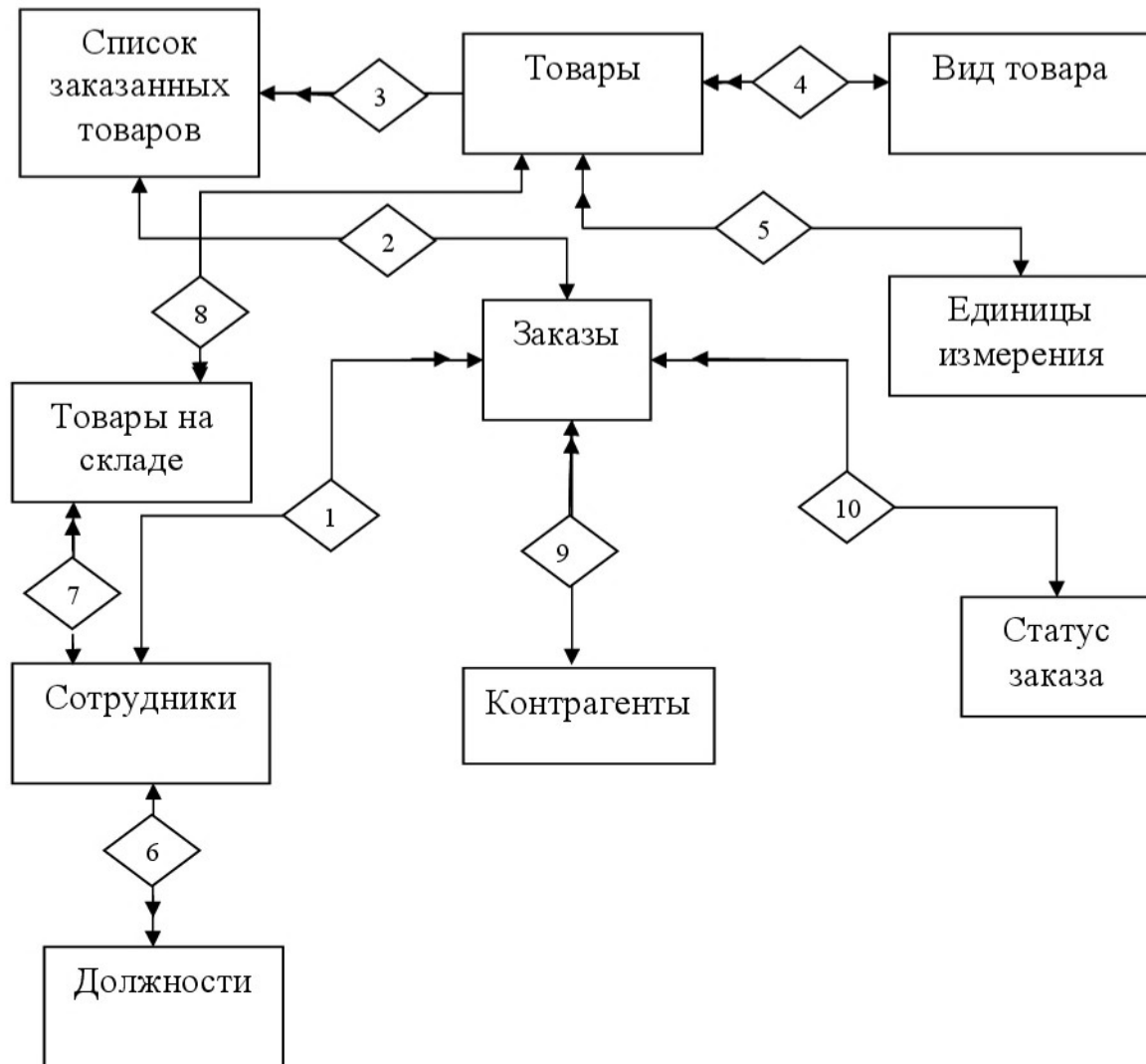
Рисунок 2.1 – Схема инфологической модели
