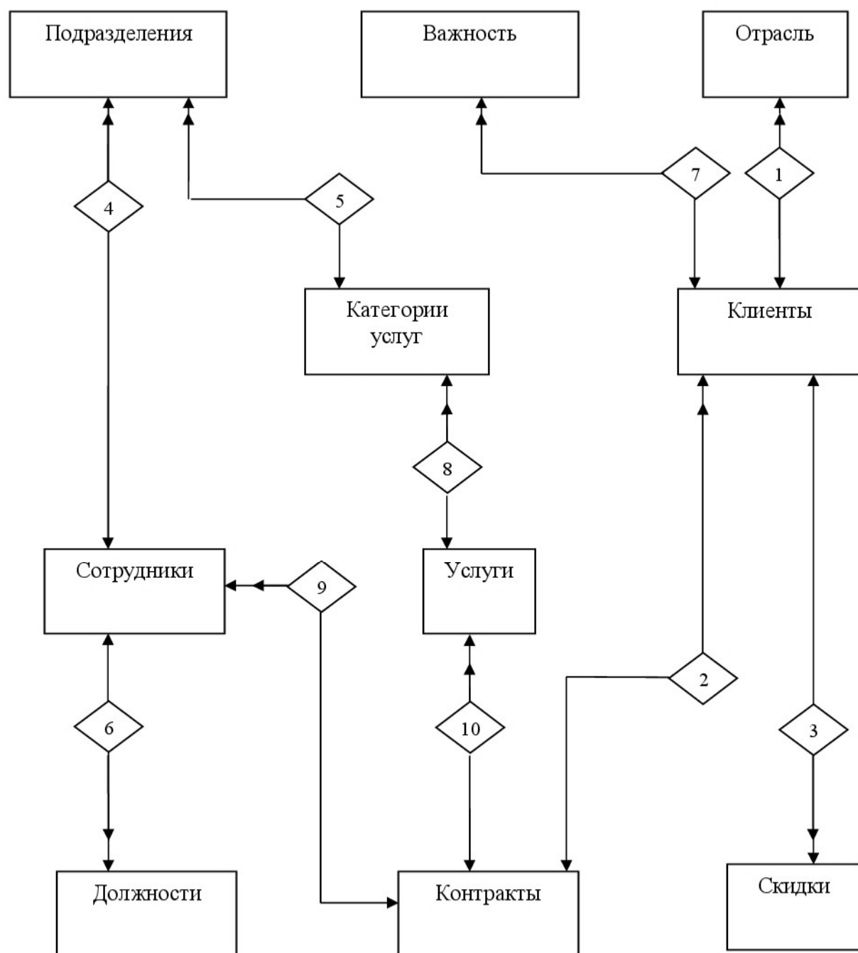
Рисунок 1.1 – Схема инфологической модели
