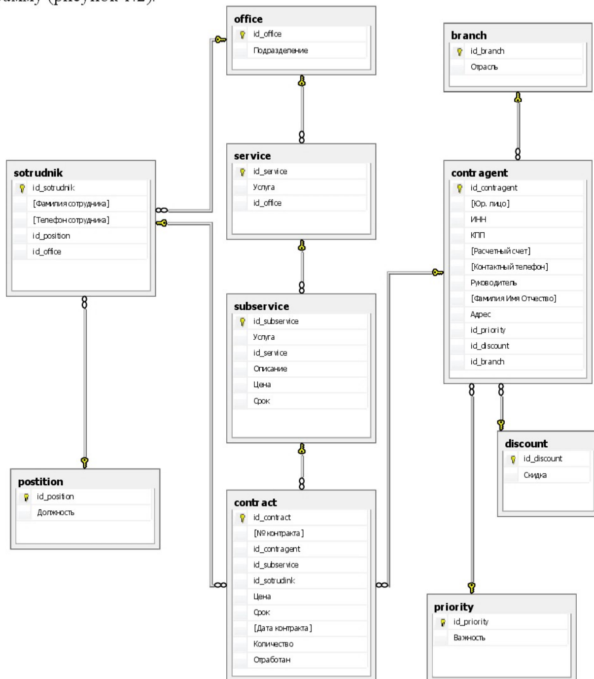
Рисунок 1.2 – ER-диаграмма
