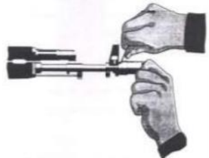
Рис. П.2.19. Отделение дульного тормоза-компенсатора
