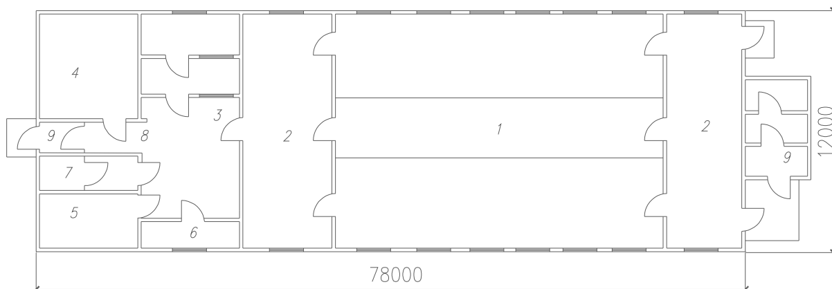
Рисунок 11-Птичник клеточного содержания на 30 тыс. кур-несушек. Вариант с деревянными трёхшарнирными арками
