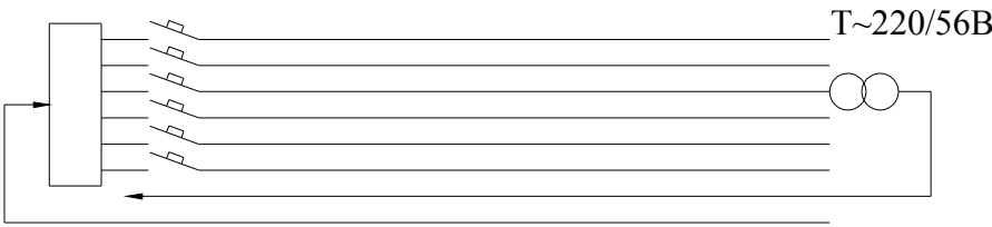
Рисунок1-Пример однолинейной электрической схемы осветительной сети
