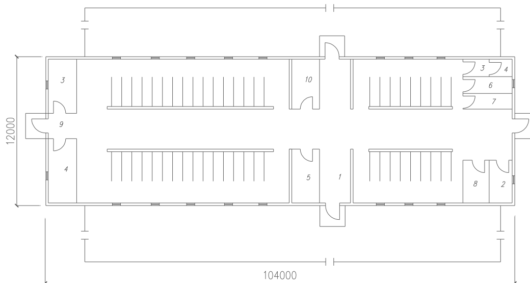
Рисунок 7- Свинарник для ремонтного молодняка на 540 мест
