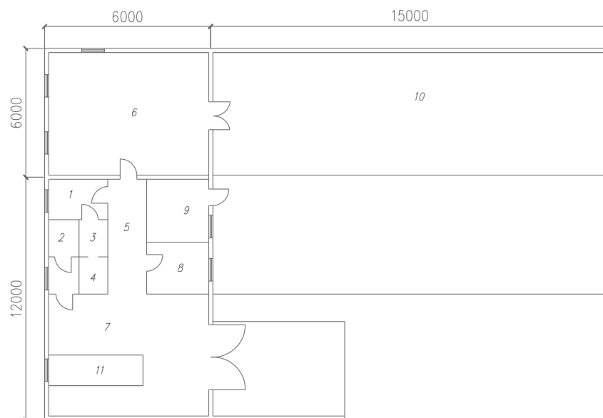
Рисунок 9- Кузница с помещением для обслуживания сельскохозяйственной техники бригады
