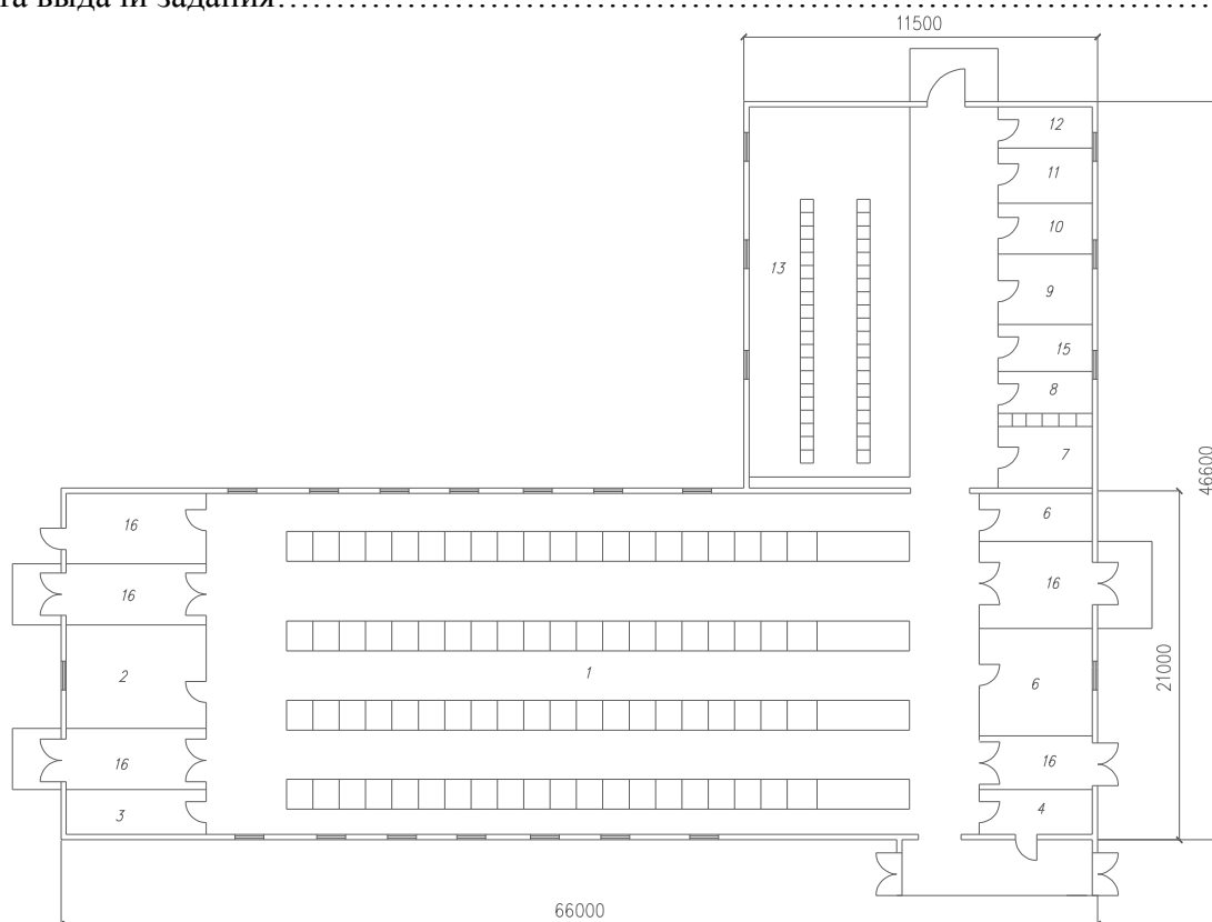
Рисунок 10- Родильная на 160 коров
