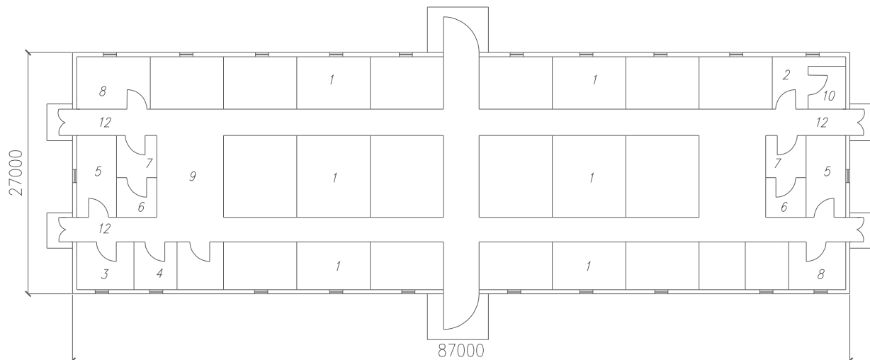
Рисунок 8- Телятник на 520 голов
