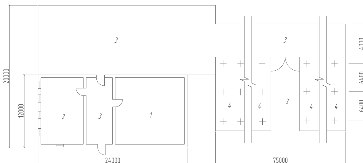
Рисунок4-Блок зимних теплиц. Рассадное отделение и энергетический пункт
