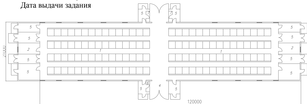
Рисунок5-Коровник на 400 коров
