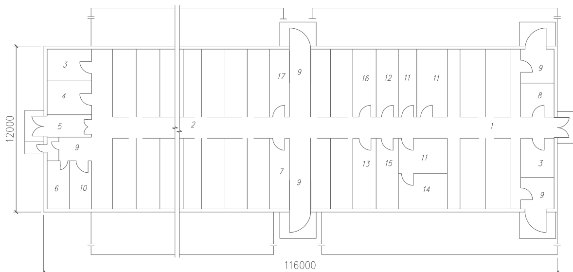
Рисунок 13-Свинарник для содержания 280 холостых маток и 10 хряков с пунктом искусственного осеменения
