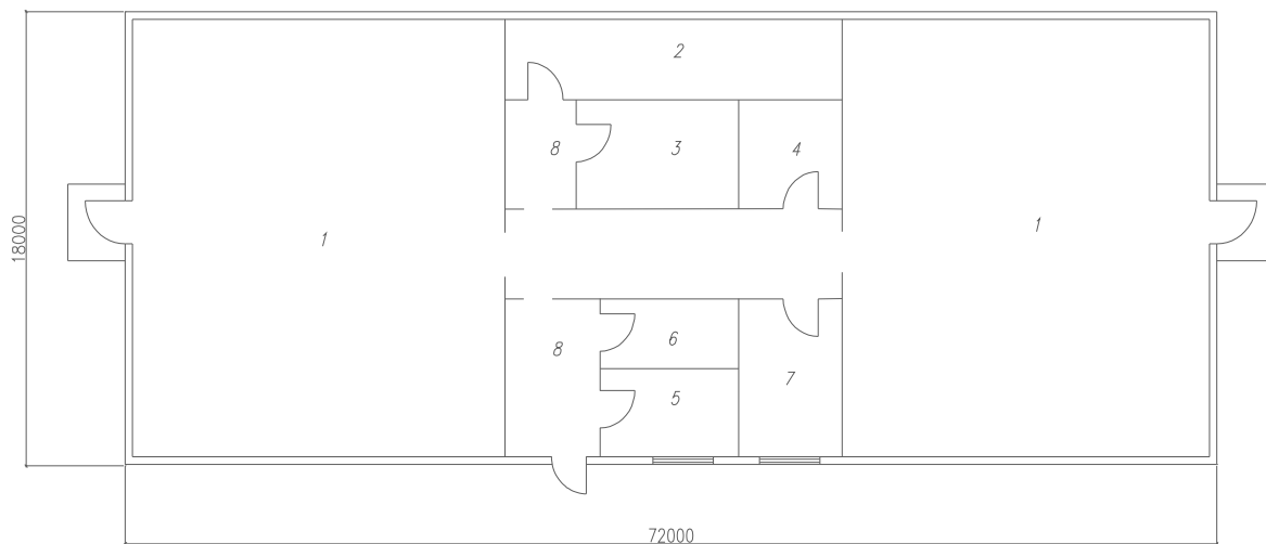
Рисунок 6-Птичник на 2500 кур яичных пород родительского и прародительского стада. Вариант с облегчёнными конструкциями ( стены из асбестоцементных панелей)
