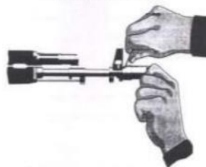
Рис. П.2.19. Отделение дульного тормоза-компенсатора
