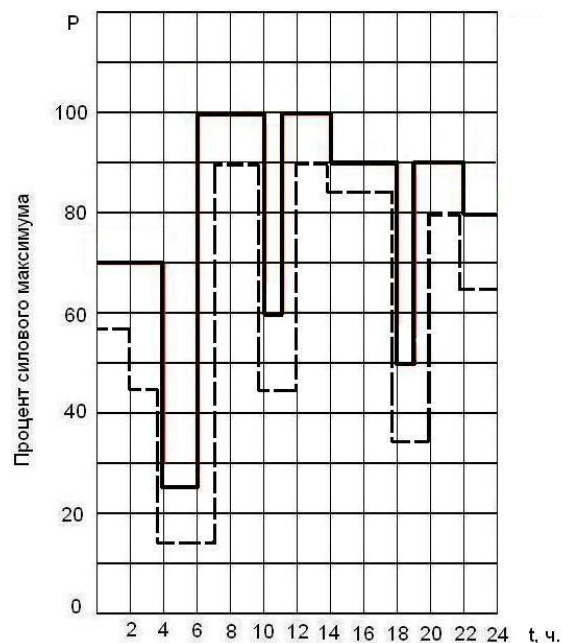
Рисунок А4 – Суточный график нагрузки бумажной промышленности _____ зима, ----- лето
