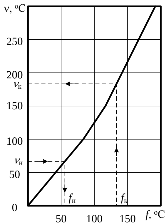
Рисунок И1 – Расчет температуры нагрева проводника
