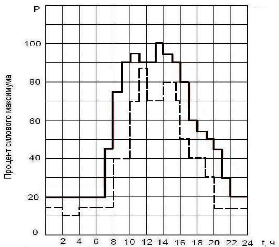
Рисунок А1 – Суточный график нагрузки с.-х. района _____ зима, ----- лето
