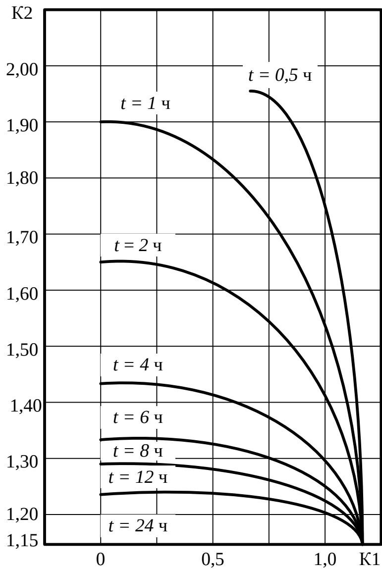
Рисунок Д1– График перегрузочной способности трансформатора системы охлаждения Д, мощностью 6,3...32 МВА, \nu_{\text{охл.}} = 0 °С
