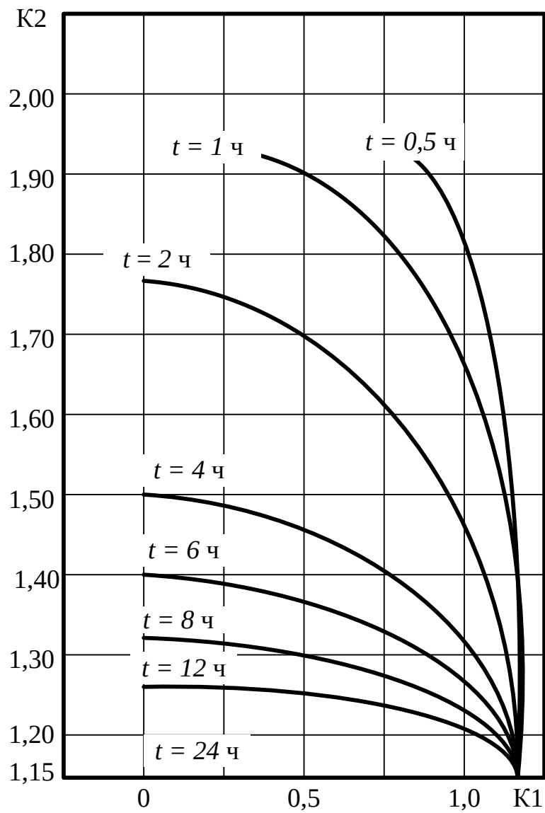
Рисунок Д2 – Кривые перегрузочной способности трансформатора системы охлаждения Д, мощностью 32...63 МВА, v_{\text{охл.}} = 0 °С
