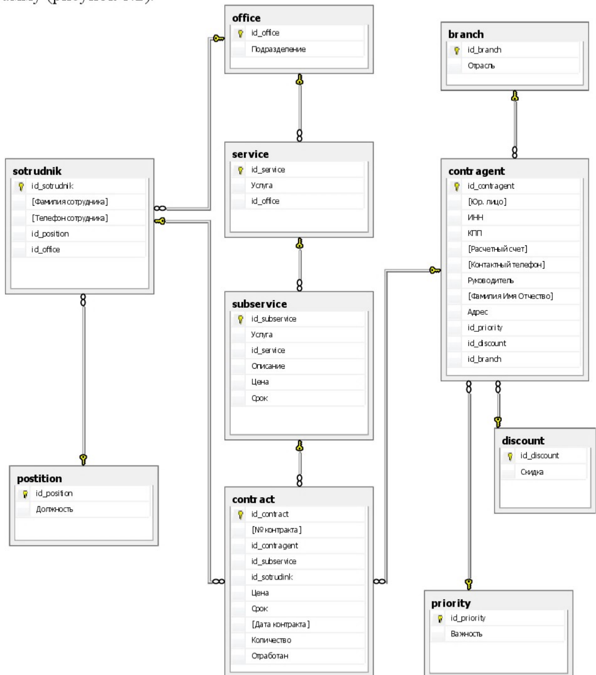
Рисунок 1.2 – ER-диаграмма
