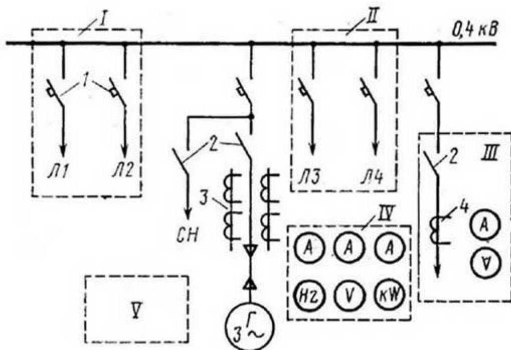
Схема типовой дизельной электростанции напряжением 0,4 кВ с одним генератором: I, II — блоки отходящих линий, III — блок ввода сети, IV — панель управления, V — блок регулирования напряжения; 1 — автоматические выключатели, 2 — рубильники, 3 — трансформаторы тока генератора, 4 — трансформаторы тока ввода сети; CH — собственные нужды, Л1–Л4 — отходящие линии
