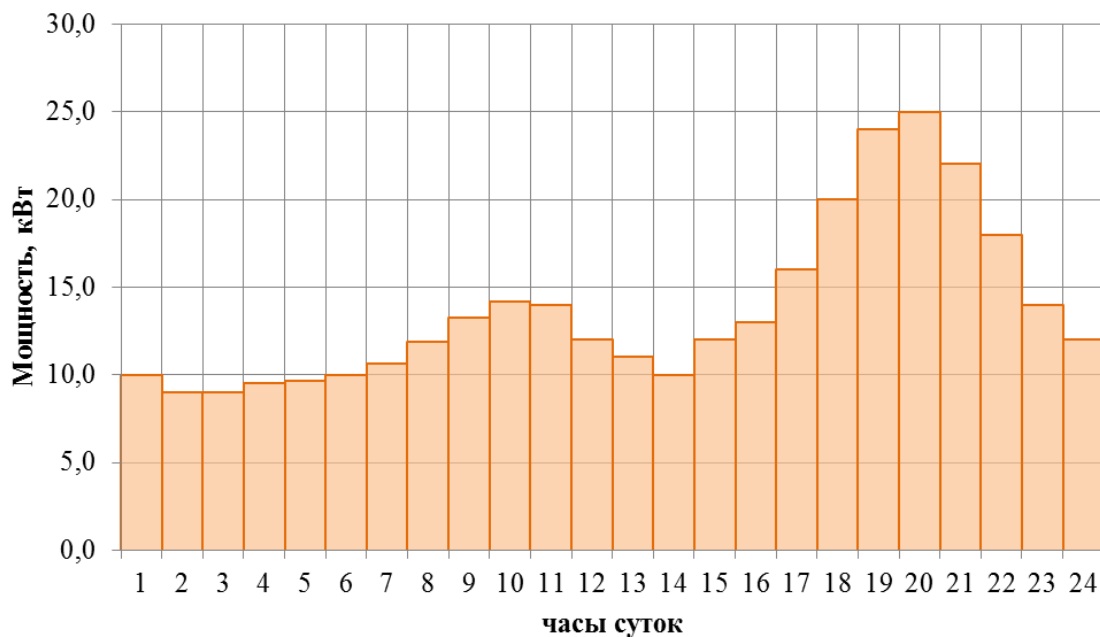
Рис. 4. Суточный график нагрузки децентрализованного потребителя
