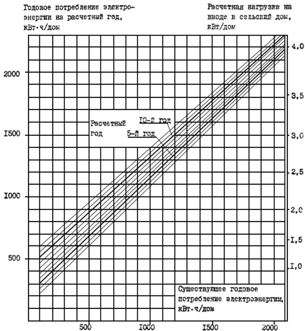
Рис.2. Удельная расчетная нагрузка на вводе в сельский дом и перспективное потребление
