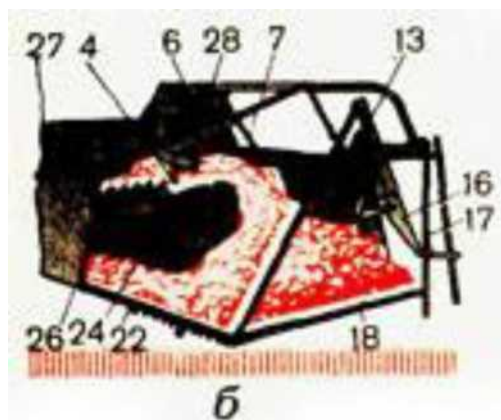
б, в- схема рабочего процесса заполнения копнителя и выгрузки
