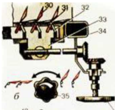
б - механизм регулирования открытия жалюзи решет;
