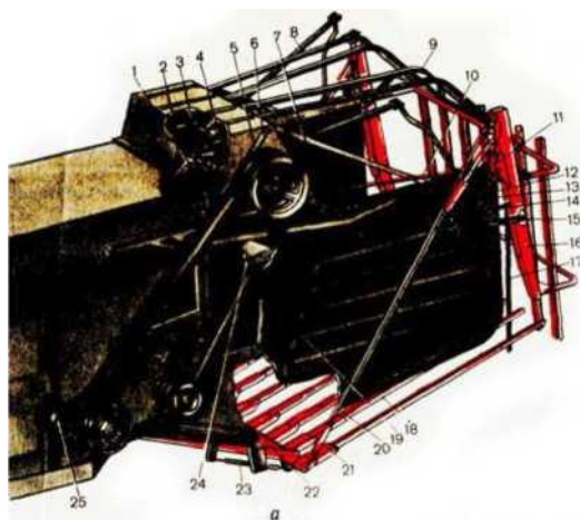
Рис. 13. Копнитель: а- общий
