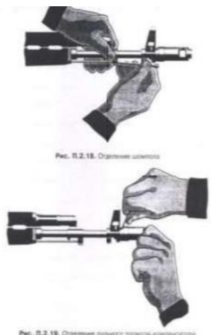
Рис. П.2.19. Отделение дульного тормоза-компенсатора
