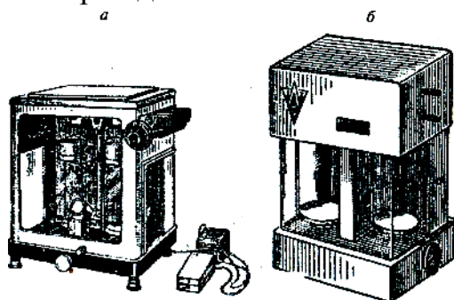
Рис. 12. Аналитические весы: а - АДВ-200; б - ВЛР-200
