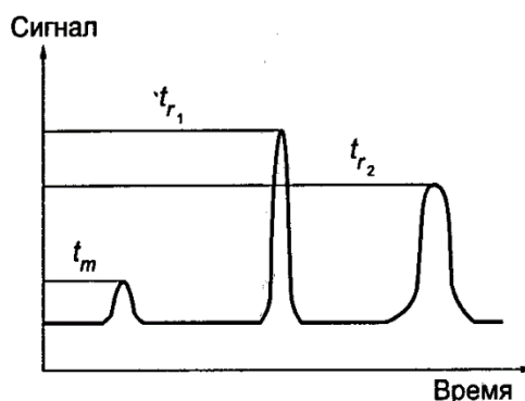
Рисунок 1 - Хроматограмма смеси двух веществ: r_1 , r_2 , m – компоненты
