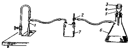
Рис. 4 Фильтрация через стеклянный фильтрующий тигель
