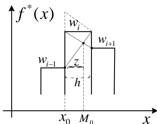
Рисунок 2.2 - К определению моды M_0
