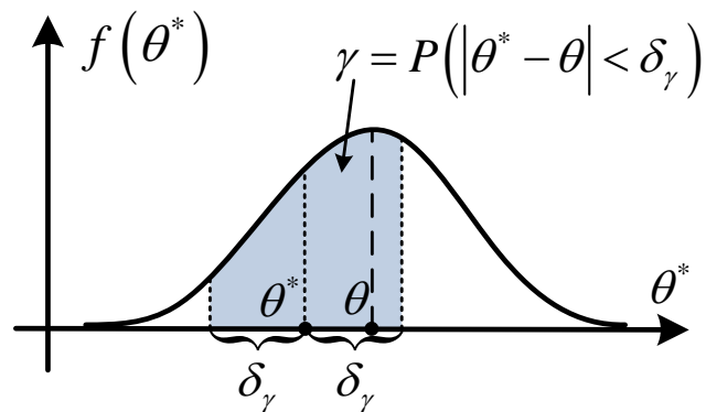
Рисунок 2.3 - К определению интервальной оценки \theta^*
