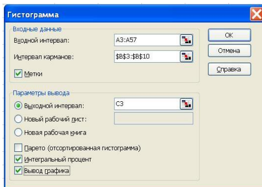
Рисунок 1.3 - Диалоговое окно режима Гистограмма
