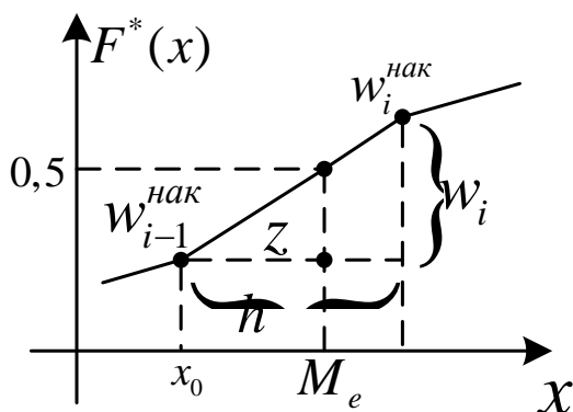
Рисунок 2.1 - К определению медианы M_e
