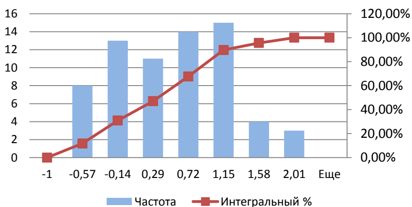
Рисунок 1.4 - График построенной гистограммы
