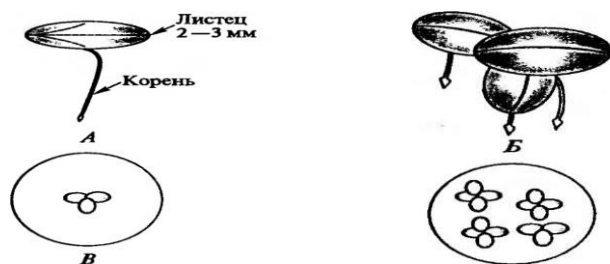
Рисунок 1 – Строение Lemna minor L. (Л. В. Цаценко, Н. Г. Малюга, 2009)
